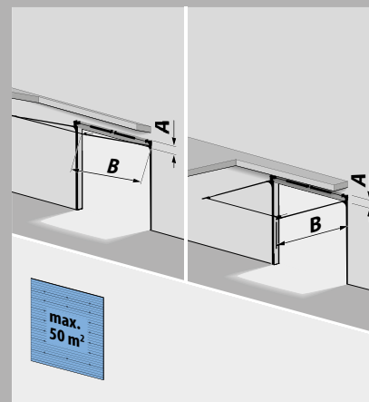
T 450 (B45), standard skinneresystem (er standard)
