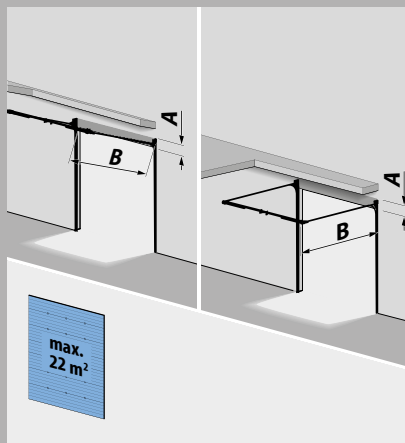
T 340 (B34), standard skinneresystem, ophængspakke bag + stålstøtteprofil
