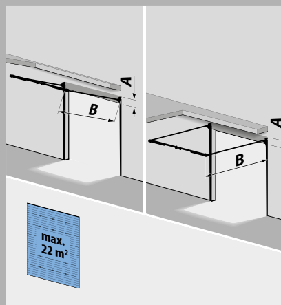
T 240 (B24), lavt løft skinneresystem, integrerede kabler + stålstøtteprofil
