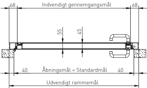
Vandret sektion/ installation bag åbningen
