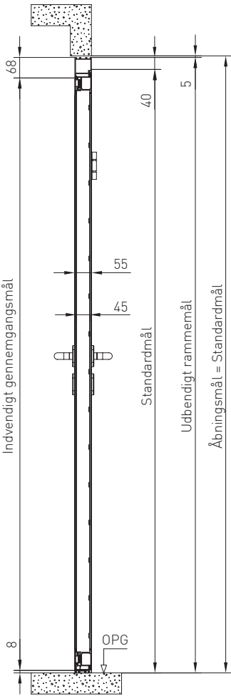
Lodret snit/installation i åbningen
