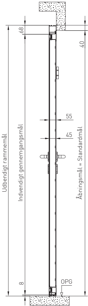
Lodret sektion/ installation bag åbningen
