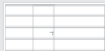
Asymmetrisk arrangement for portbredde BRB 3.501 - 4.250 mm - til venstre eller højre fra midten af porten
