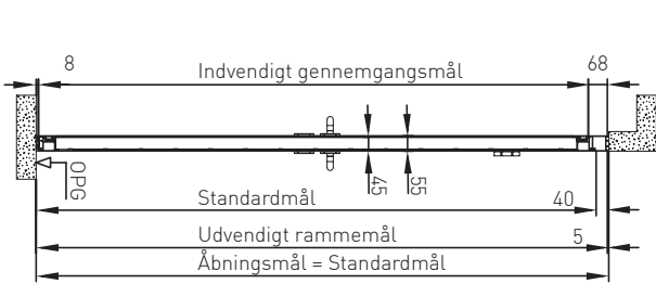
Vandret sektion/ installation i åbningen
