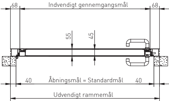
Vandret snit/ indbygning bag åbningen
