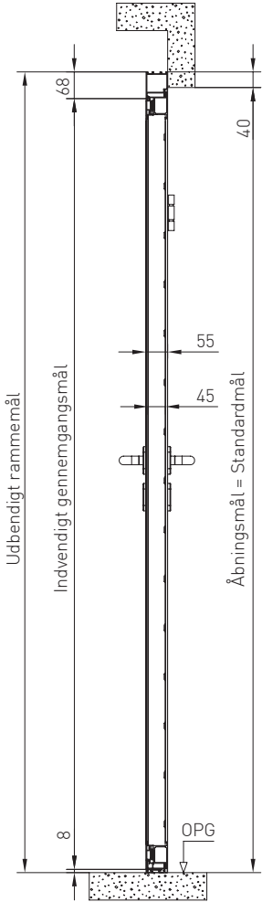
Lodret snit/ indbygning bag åbningen
