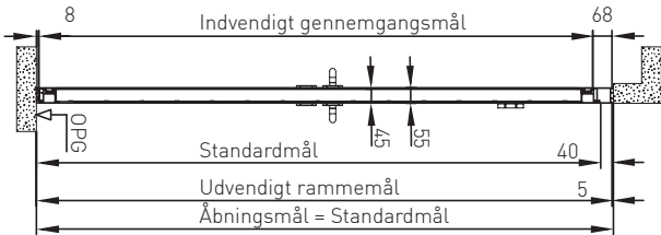
Vandret snit/ indbygning i åbningen
