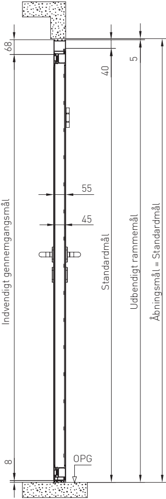
Lodret snit/ ndbygning i åbningen
