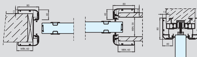
Sektion med skydedørsplade inde i væg.
