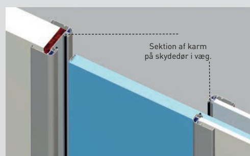
Sektion med skydedørsplade inde i væg.
