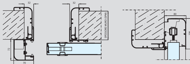
Sektion med med skydedør uden på væg.
