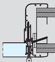
Montering på gipsvæg.
