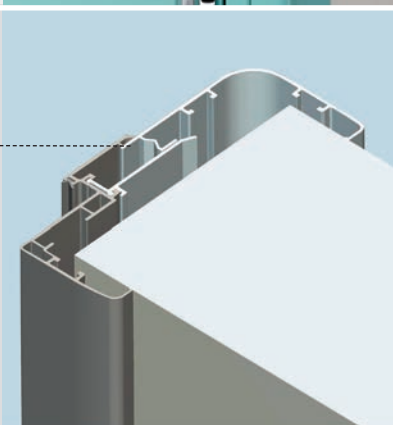
Sektion med omsluttende karm, forlænget med mm 60.
