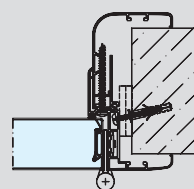
Montering på massiv væg.
